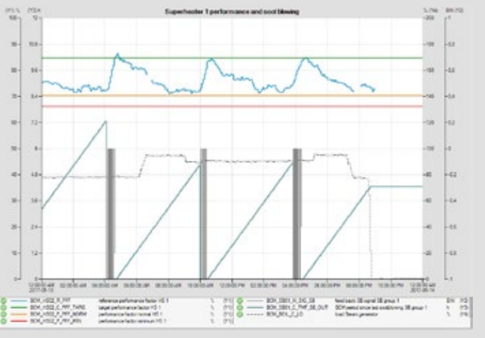
Verschmutzungstrend
